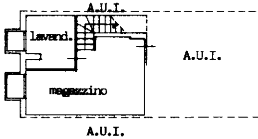
PIANO PRIMO SOTTOSTRADA H = 2,50 mt.
