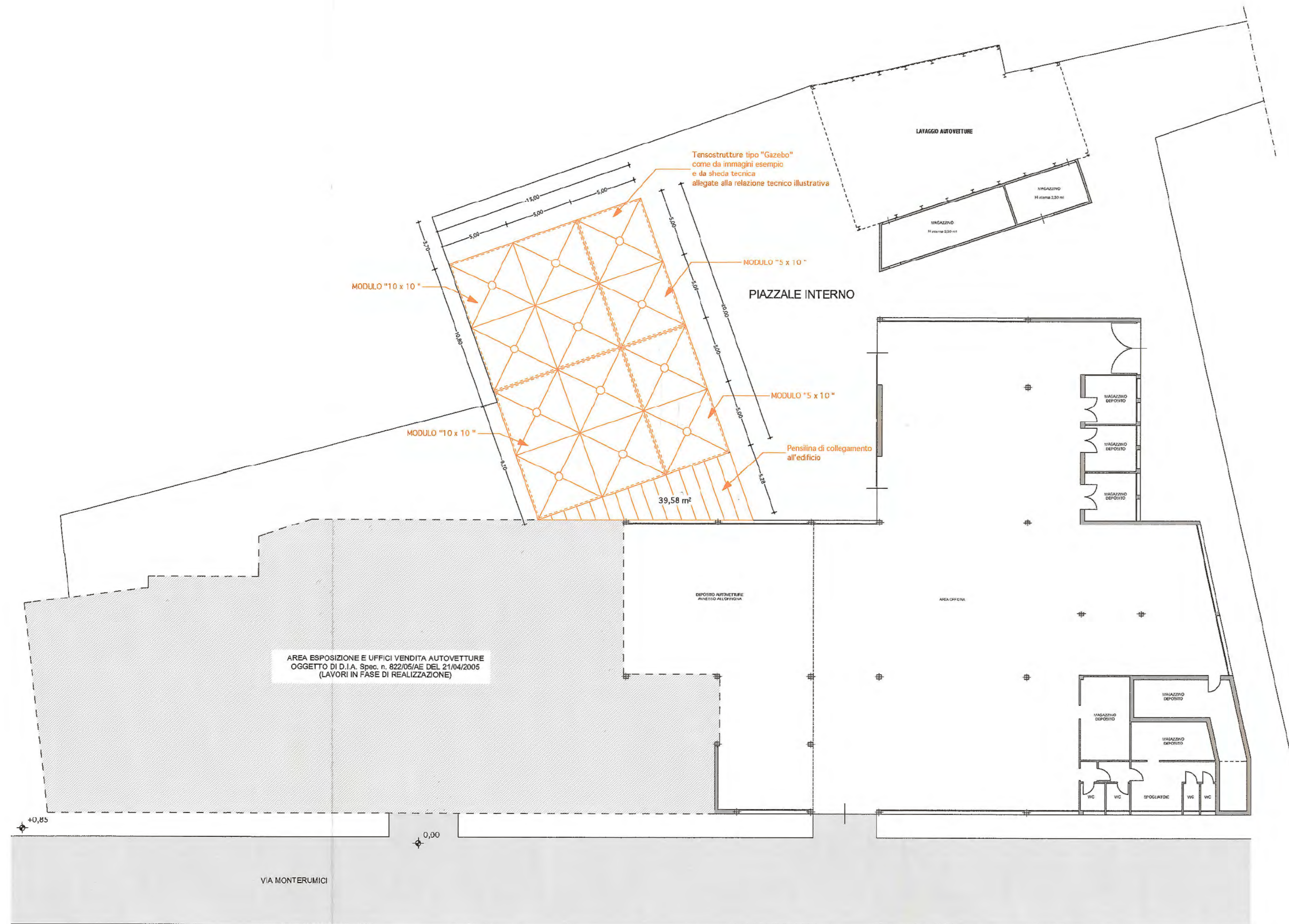
PIANTA PIANO TERRA - 1:200
